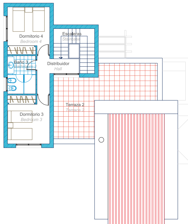
Planta Alta / Top Floor
